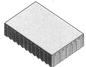
Topline BVS 59,6 x 39,6 x 10,8 cm
