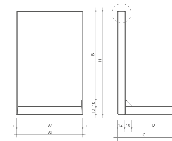
TYP 2 Höhen 130 - 155 cm
