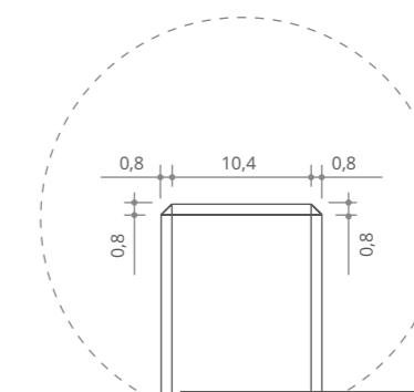
kleine umlaufende Fase 0,8 x 0,8 cm
