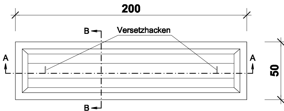
Draufsicht Maßstab 1:200
