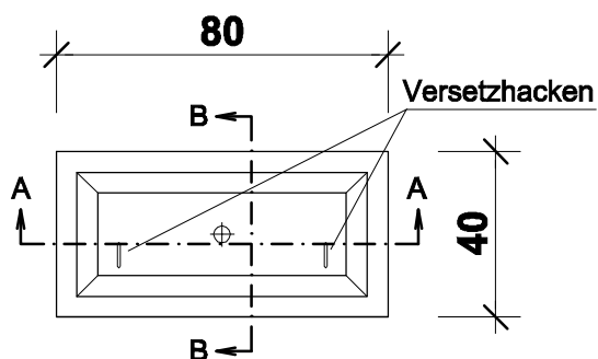
Draufsicht Maßstab 1:200
