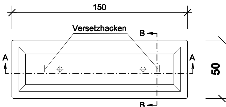
Draufsicht Maßstab 1:200
